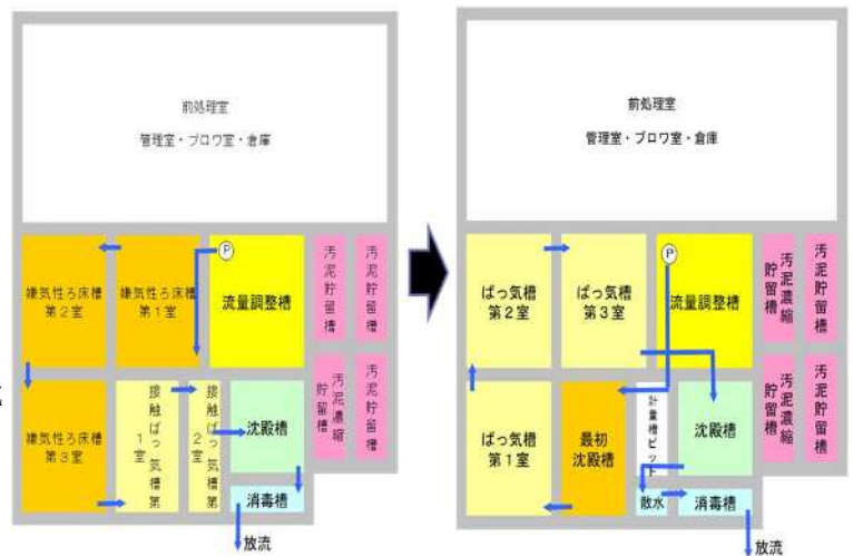
処理方式の切替え改築のイメージ (生物膜方式JARUS-III型→浮遊生物方式JARUS-XIV R 型)
