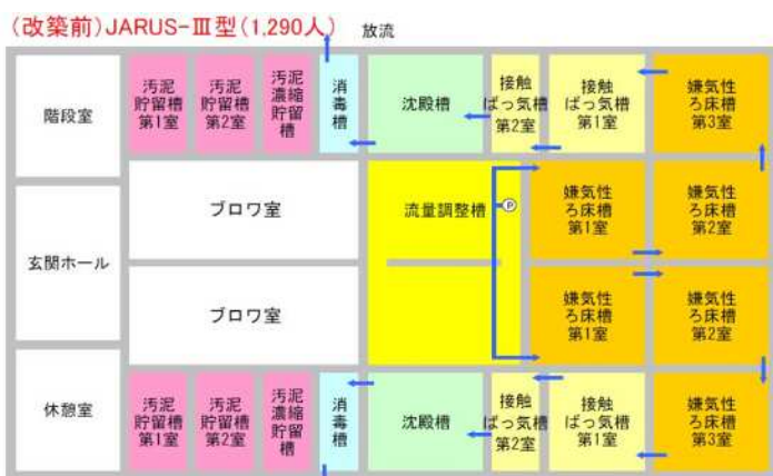
改築前（JARUS-III型）
