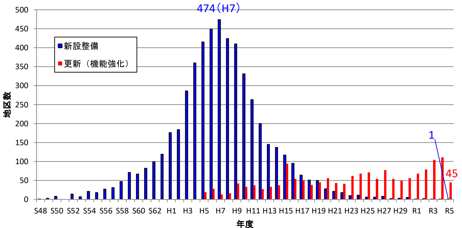
農業集落排水施設(採択地区数)の推移
