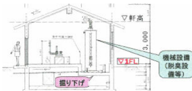
図 11-2 床面掘り下げによる軒高の抑制
