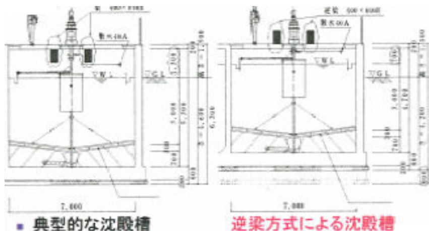
図 11-1 逆梁方式による沈殿槽
