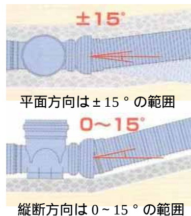
図参 1-3 角度調整が容易なリブ付小型マンホール（例）
